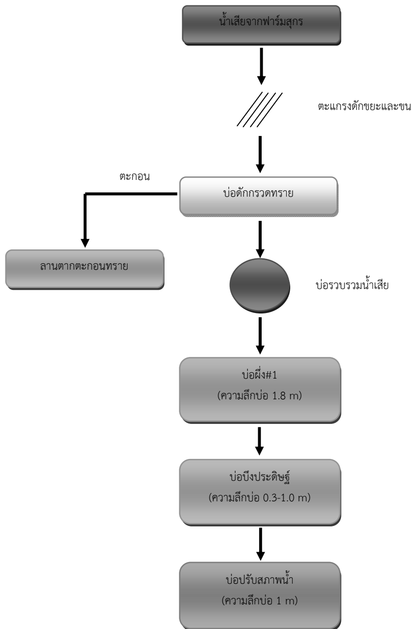
รูปที่ 6.4-4 กระบวนการบำบัดน้ำเสียแบบบ่อฝั้แบบผสม
